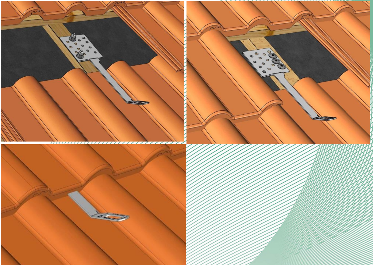
Bilder 1 - 3: Anschlageinrichtung, Typ: LUX-top® SDA-Z II (Montagebeispiele)
